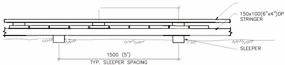
SIDE ELEVATION SCALE: 1:20
